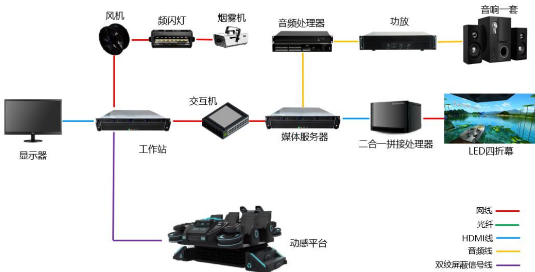
图 48 5D 影院系统拓扑图
