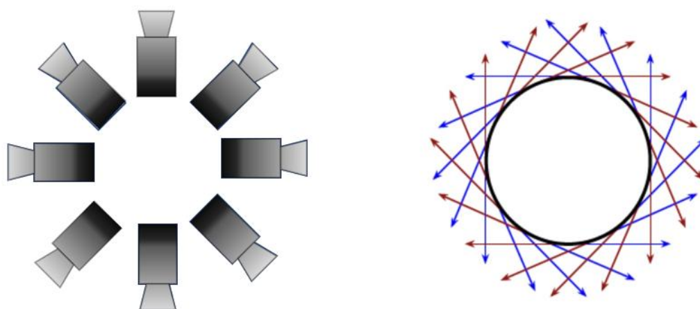
图 10 左：全景相机共光心环形排布、右：ODS 模型
