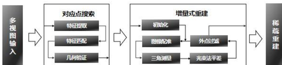
图 17 典型的 SFM 算法流程
