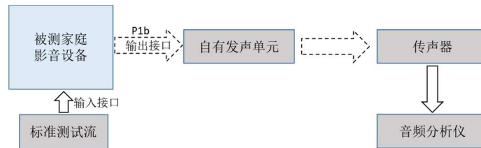
图3 声性能测试连接图 (p1b 可以不用了)
