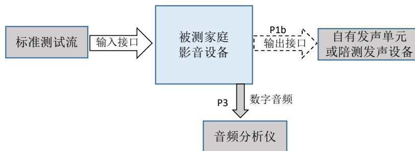
图1 解码功能测试连接图
