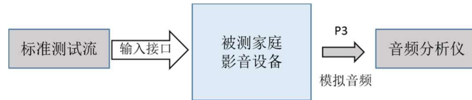
图2 电性能测试连接图
