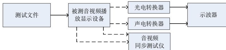
图4 音视频播放显示设备音视频同步测试框图
