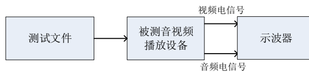
图5 音视频播放设备音视频同步测试框图
