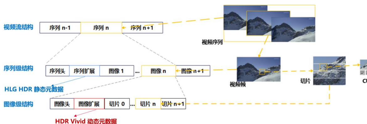
图 3 HDR Vivid 动态元数据在 ES 码流中的封装示意
