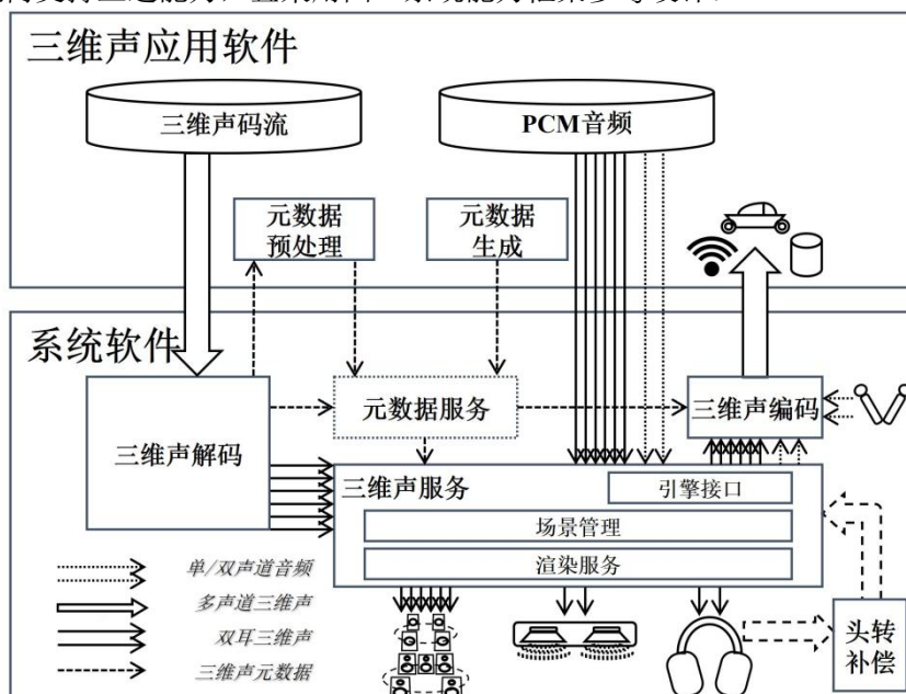
图 1 智能终端三维声系统能力框架参考设计
