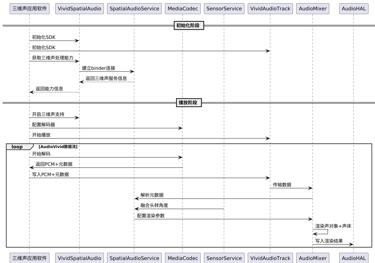
图 5 正常播放流程示例
