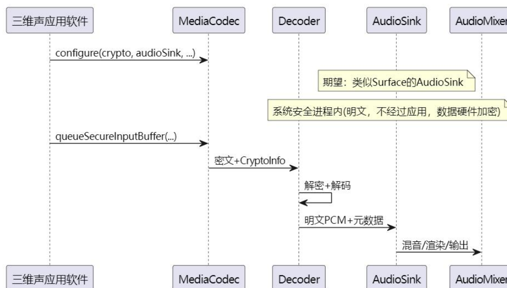
图 A. 3 DRM 流程示例（期望方案）
