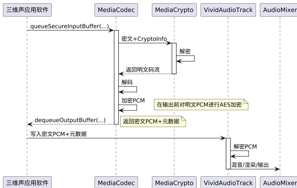
图 A. 2 DRM 流程示例 (MediaCodec 二次加密)
