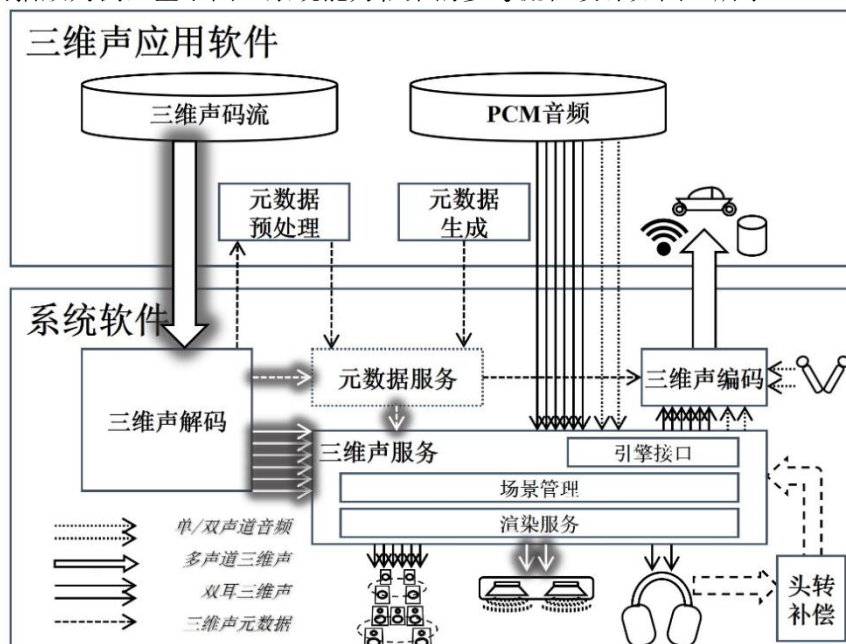
图 2 系统解码播放参考流程设计示例
