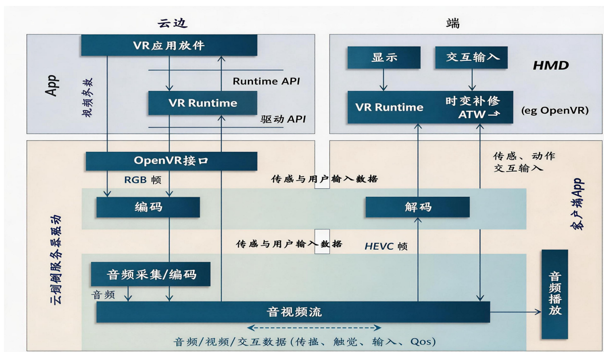
图6 云化XR解决方案架构
