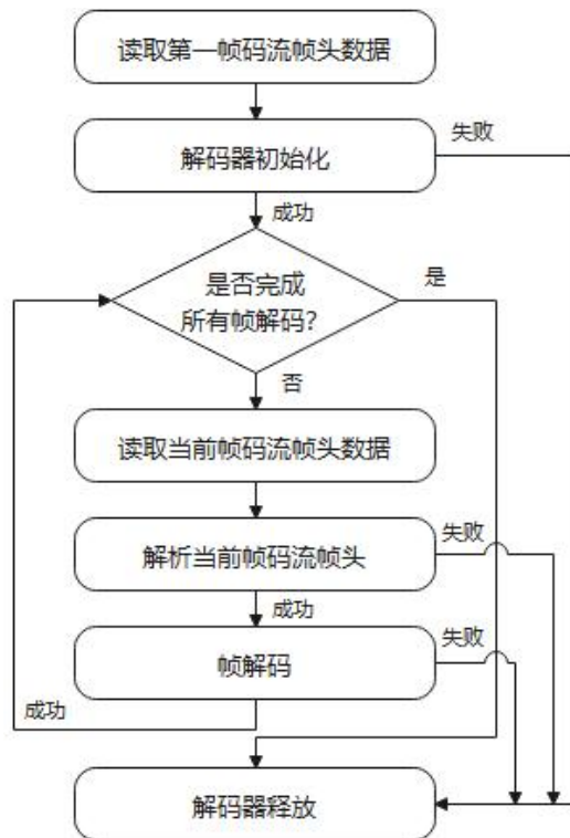
图 3 解码器 API 调用流程图
