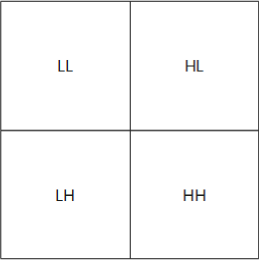
图3 小波分解结构
