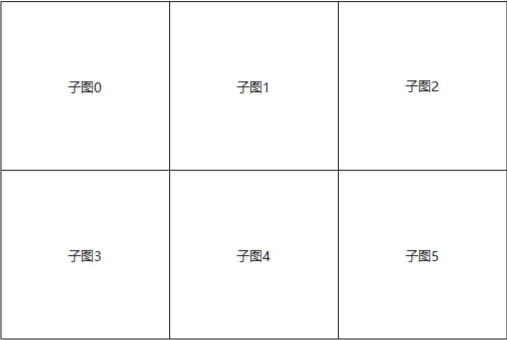
图2 子图结构
