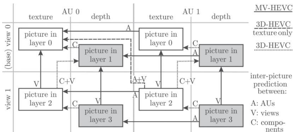
图8 MV-HEVC/3D-HEVC格式示意图
