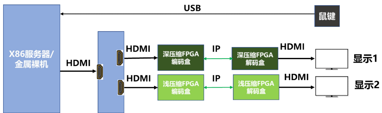
图 6 浅压缩试验样机对比测试环境
