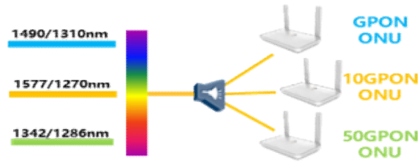
图 12 50GPON 支持局端设备多模共存
