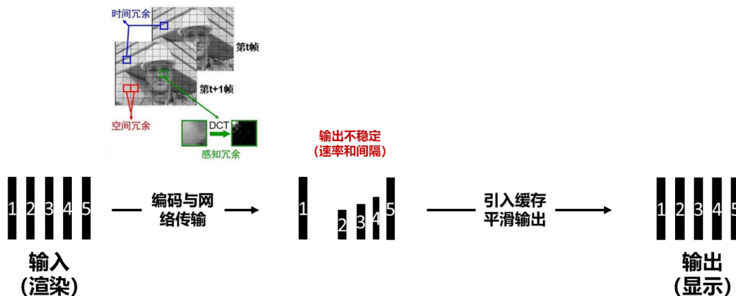
图5 深压缩编解码与传输系统示意图
