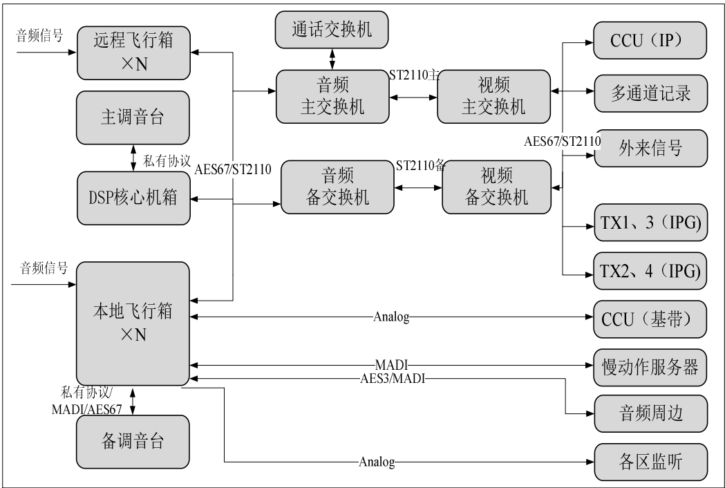
图 5 音频系统示意图
