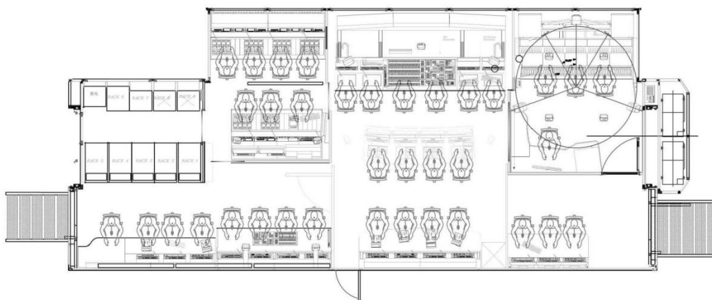
图 1 典型的 8K 超高清转播车车内布局示意图 1
