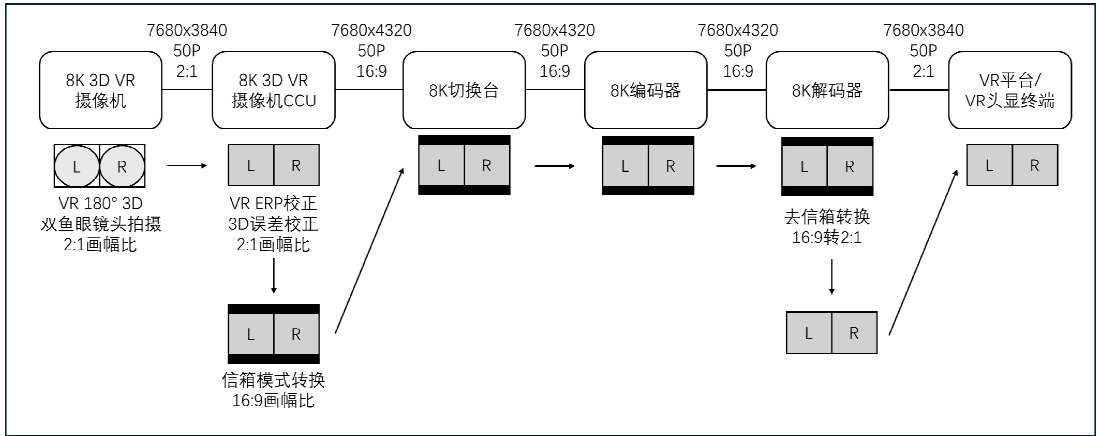
图 C1. 8K 3D VR 格式转换链路图
