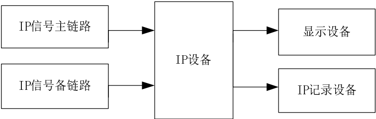
图 24 冗余备份 IP 流倒换测量框图
