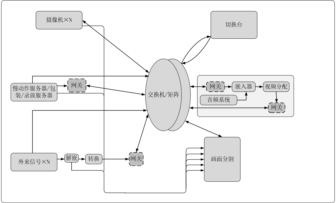
图3 以IP方式实现的视频系统示意图
