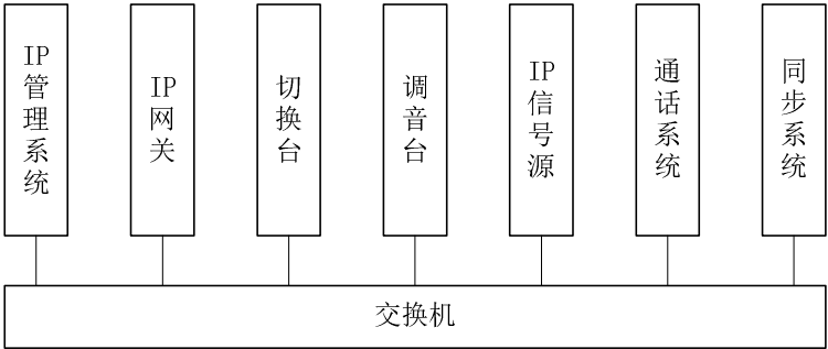
图 9 数字电视转播车典型 IP 通道
