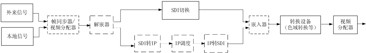
图 6 8K 超高清转播车通道（基带）示意图
