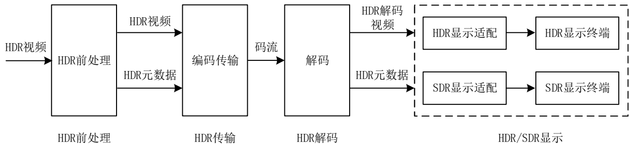
图1 带动态元数据 HDR 端到端系统
