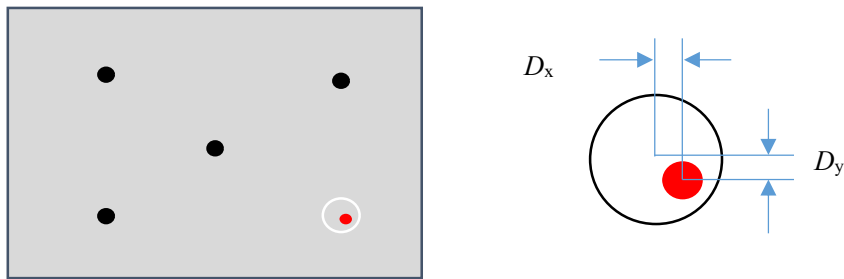
图3 位置准确度测量设置图
