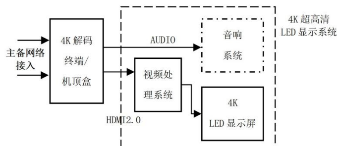
图 1 4K 超高清 LED 显示系统框图
