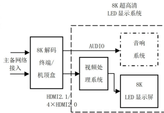
图2 8K超高清LED显示系统框图
