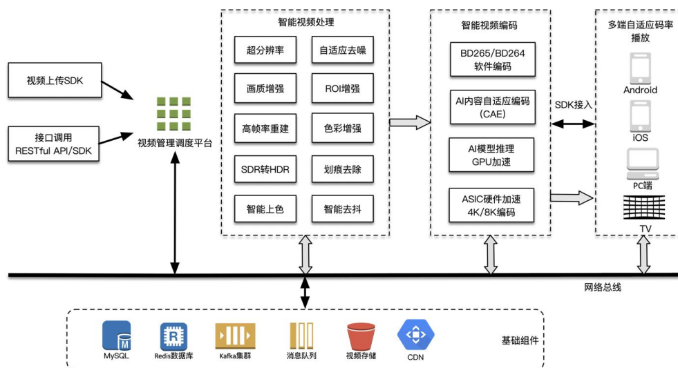
图 13 百度智能云智能超清产品架构图
