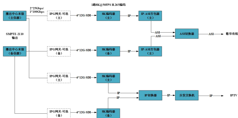
图 28 北京台 8K 频道组网图
