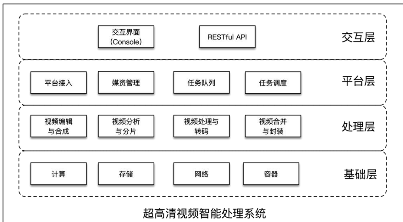
图 4 超高清视频智能处理系统技术架构
