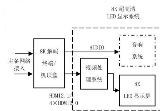
图2 8K超高清LED显示系统框图
