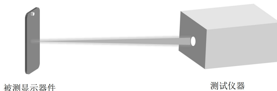
图 2 分光测色计测试方法示意图
