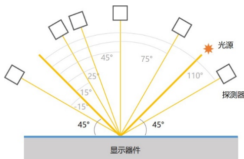
图 3 多角度色差仪测试原理示意图
