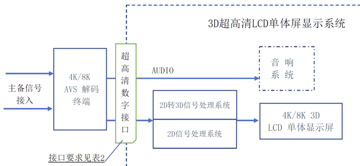
图 4 4K/8K 3D 超高清 LCD 单体屏显示系统框图
