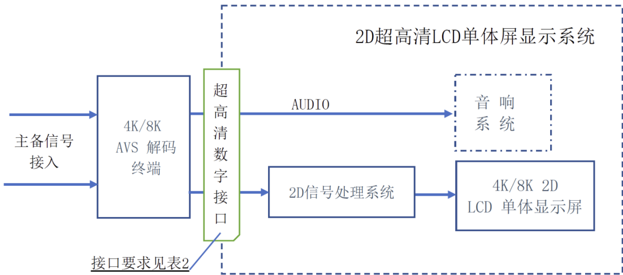
图 2 4K/8K 2D 超高清 LCD 单体屏显示系统框图
