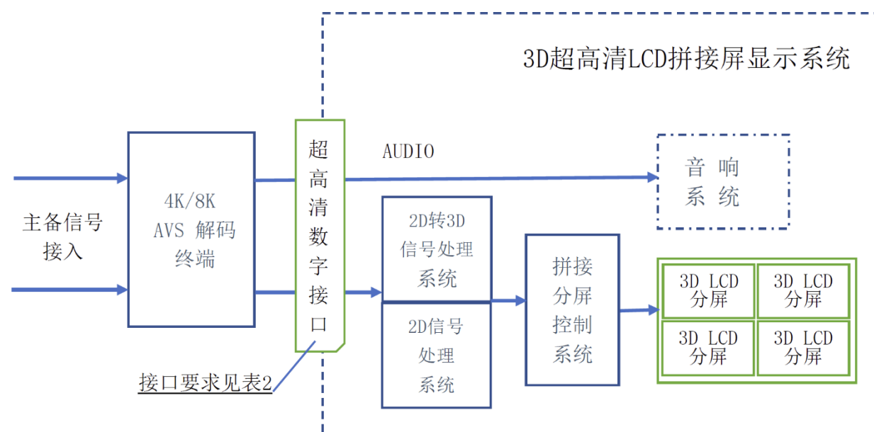
图 5 4K/8K 3D 超高清 LCD 拼接屏显示系统框图
