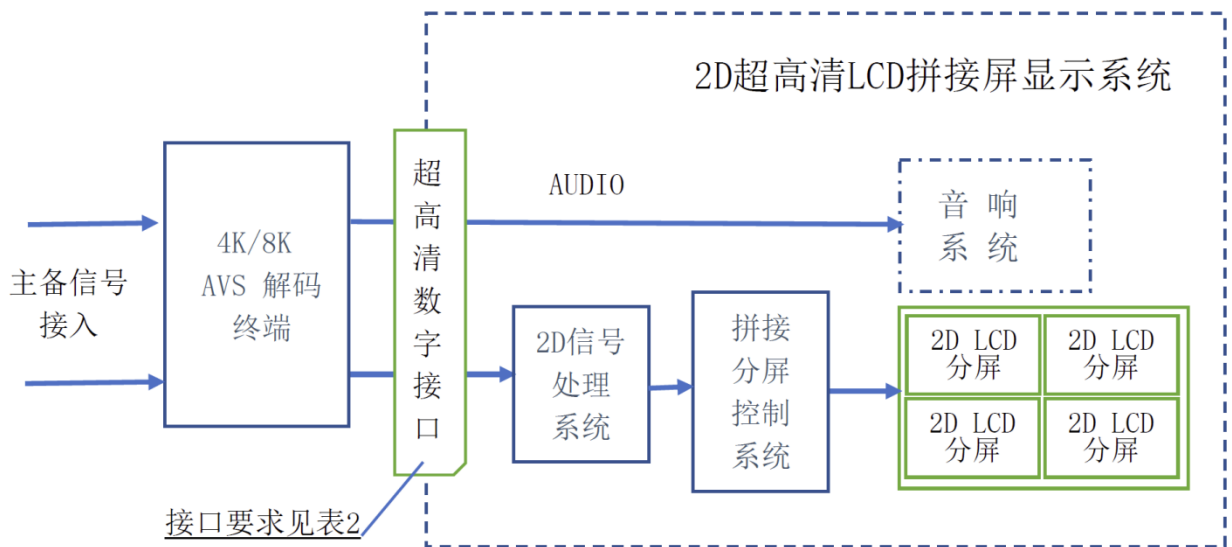
图 3 4K/8K 2D 超高清 LCD 拼接屏显示系统框图
