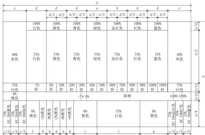
图 2 彩条信号测试图组成
